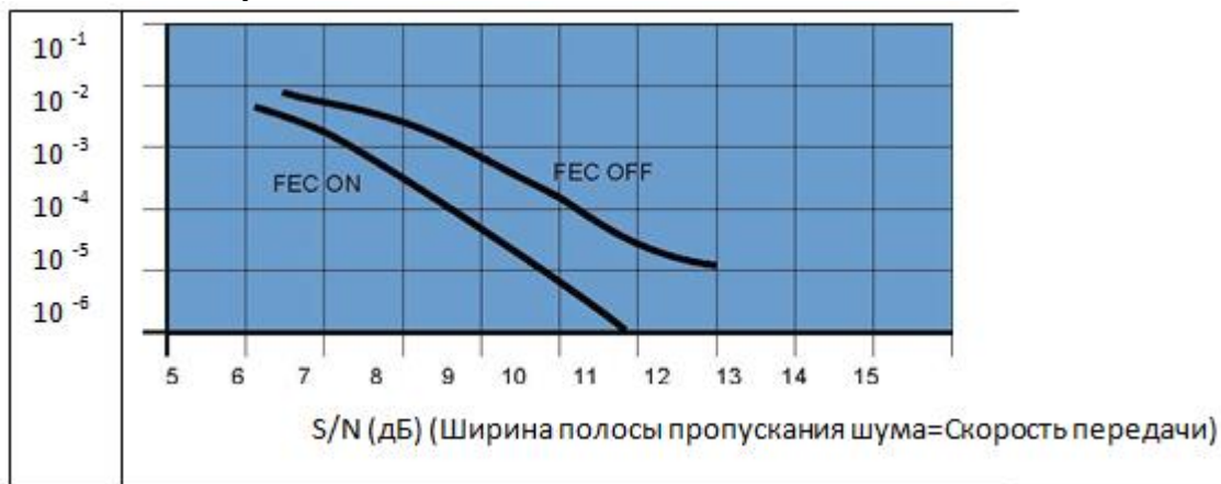
Рис. 10 – Теоретическое усиление с использованием FEC
