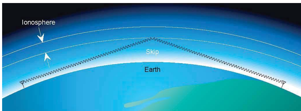
Рисунок 3. Распространение ВЧ сигнала с помощью "отражения"
