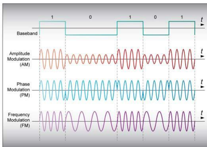
Рисунок 5. Модуляция сигнала
