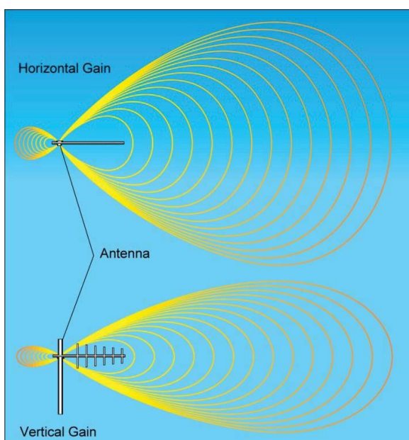
Рисунок 7. Диаграмма направленности узконаправленной антенны
