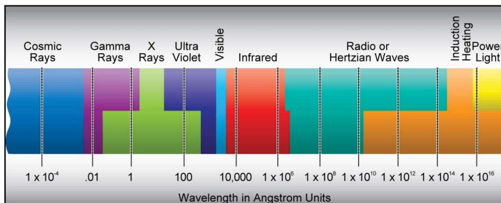
Рисунок 1. Электромагнитный спектр
